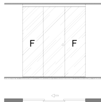
1 Door 1 Track
