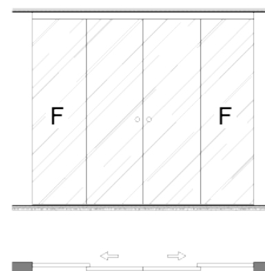
2 Door 1 Track
